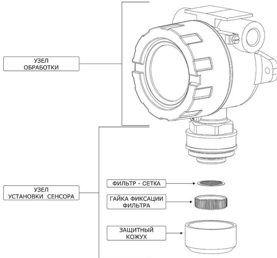
Рисунок 7 – Основной функциональный состав ИГМ-13М
