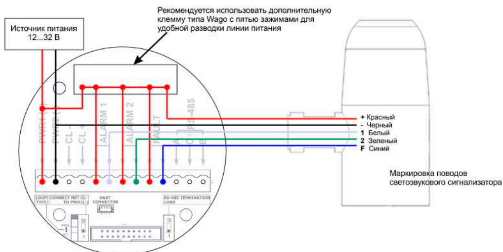
Рисунок 23 – Схема подключения светозвукового сигнализатора ЭМИ-С3 к ИГМ-13М, изготовленным с апреля 2023г.
