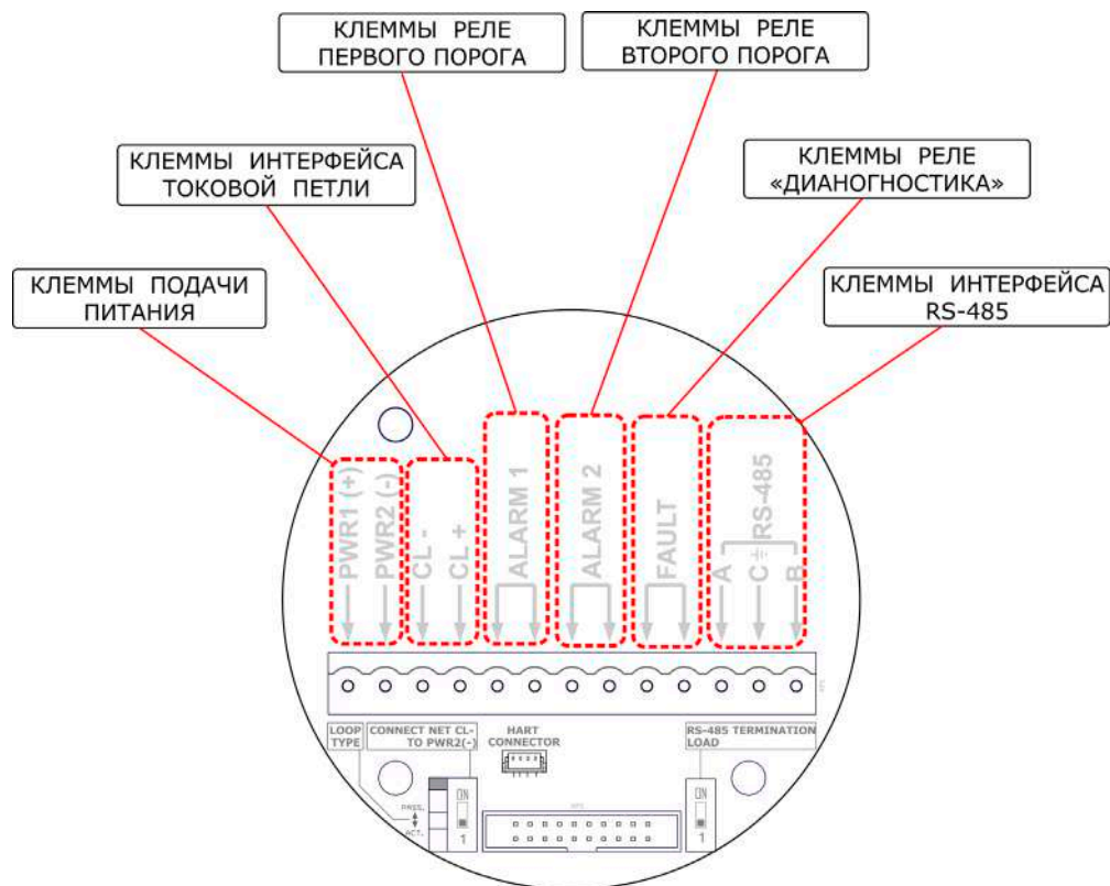
Рисунок 12 – Функциональное назначение клемм подключения внешних электрических цепей ИГМ-13М, изготовленных с апреля 2023г.
