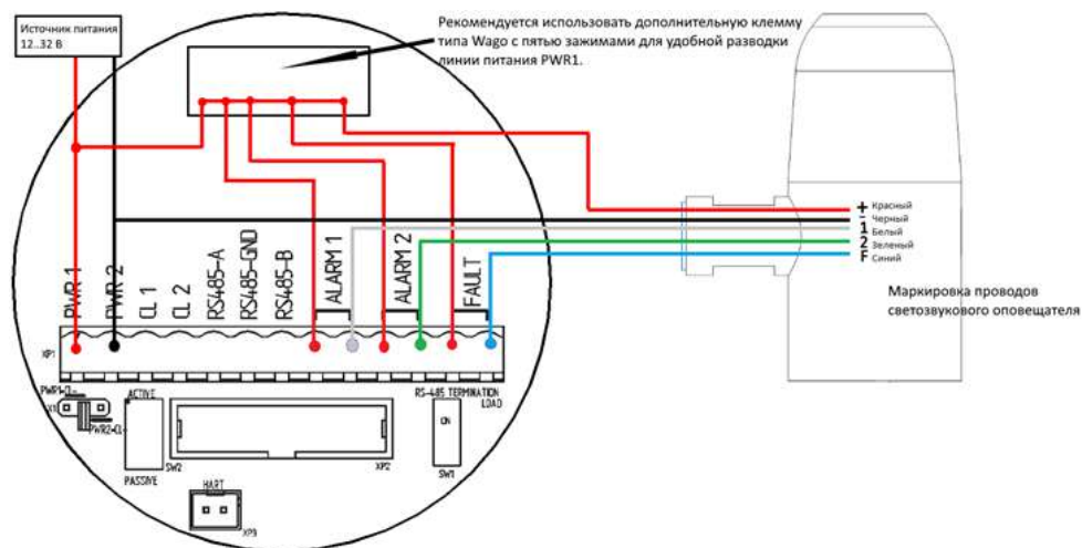
Рисунок 22 – Схема подключения светозвукового сигнализатора ЭМИ-С3 к ИГМ-13М, изготовленным до апреля 2023г.
