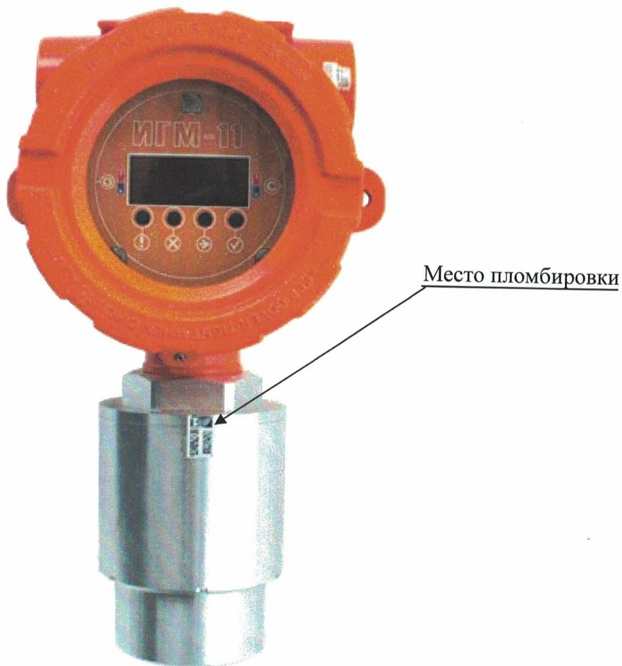
Рисунок 1 - Общий вид газоанализаторов и схема пломбировки от несанкционированного доступа ИГМ-11
